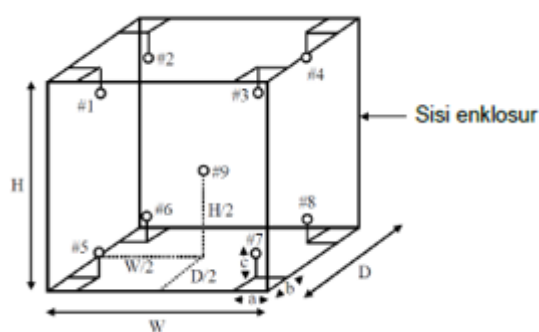
Penempatan Sensor
